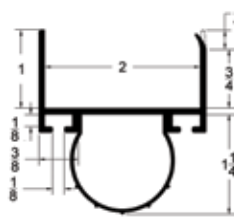
2" AR-02 ASTRAGAL
