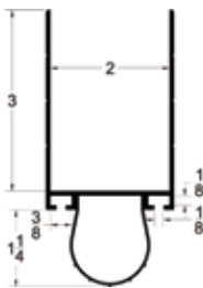
2" ARL-200
