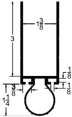
1 3/8" ARL-138
